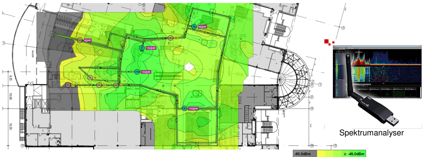
Heatmap mit Signalverlauf
